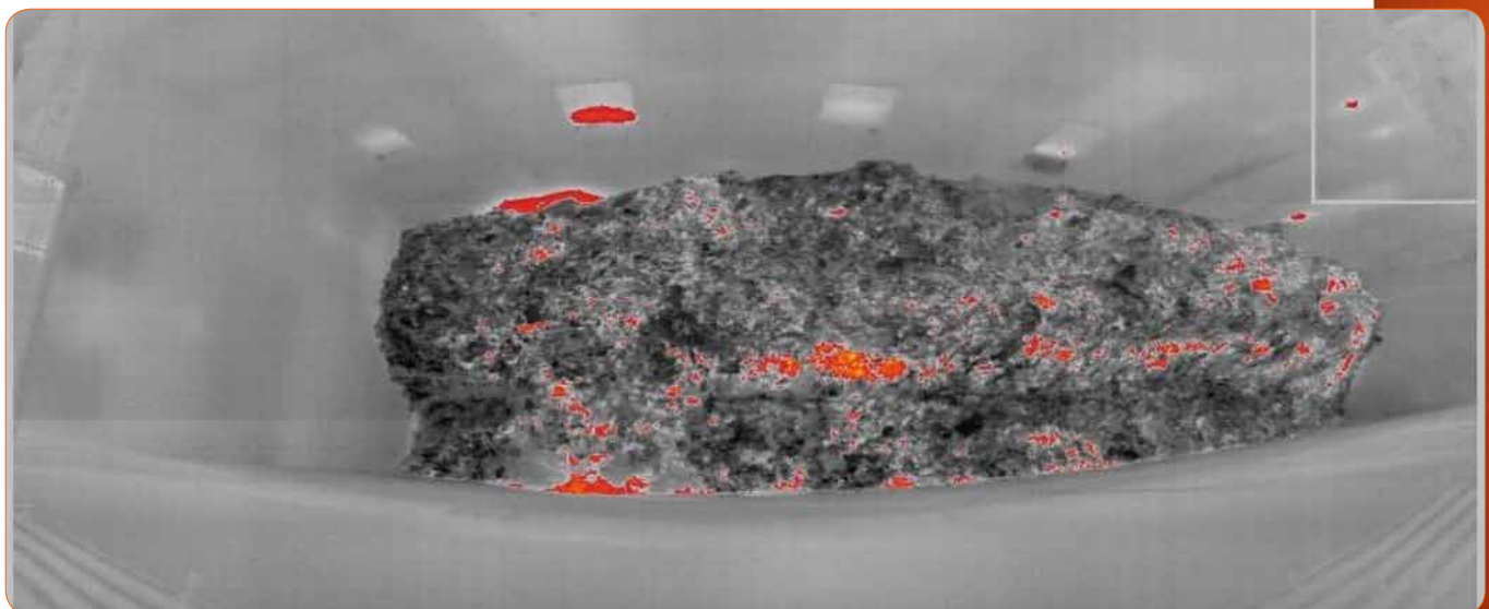
Panoramathermografie: Ansicht eines Müllbunkers mit der patentierten abiroVision® Software
