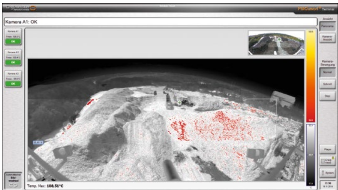
Aussenlager für zerkleinerte Reifen (230 x 100 m): Touchscreen Bedienmenü mit Darstellung der gesamten Detektionsfläche als IR-Panoramabild
